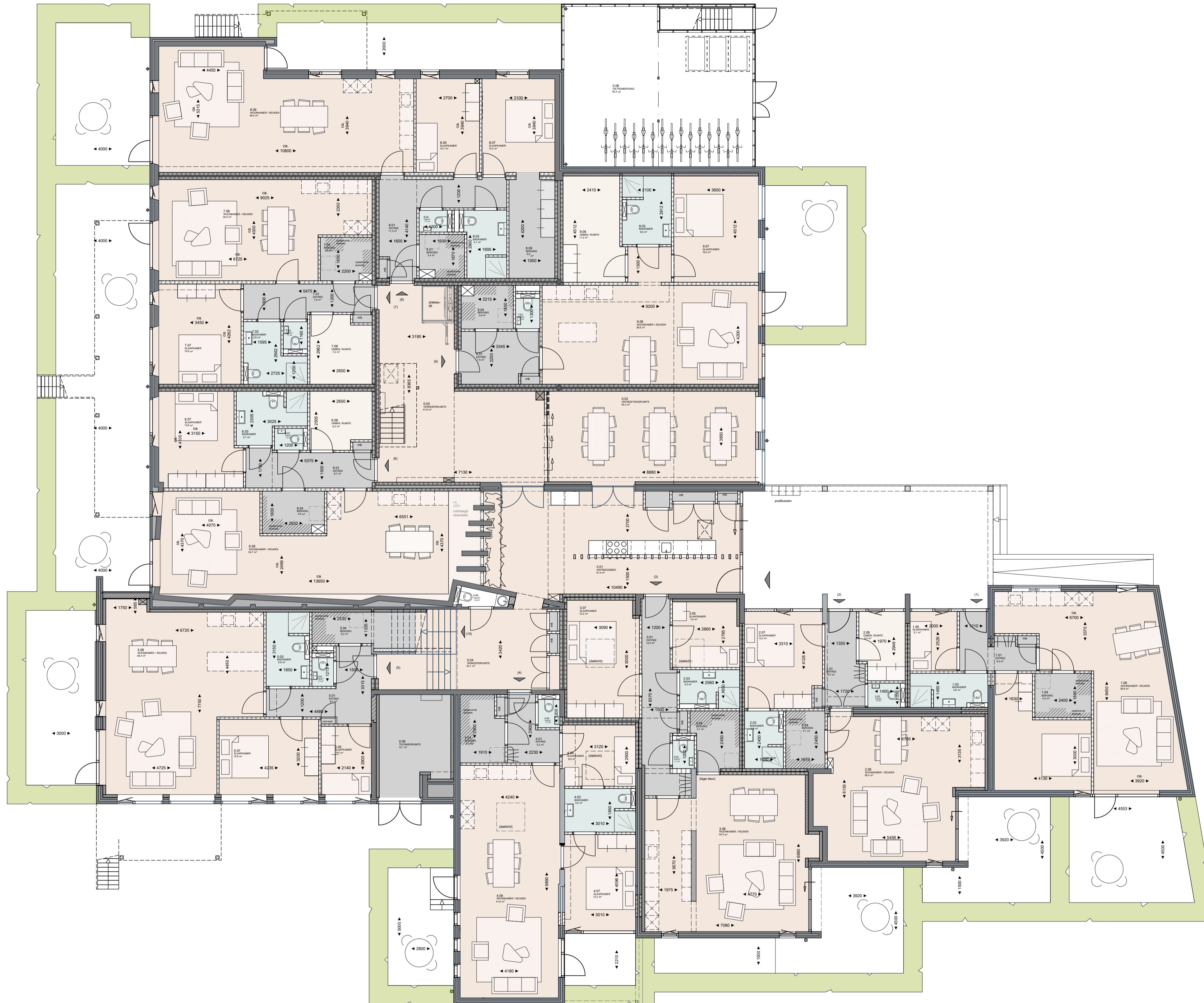
BEGANE GROND
